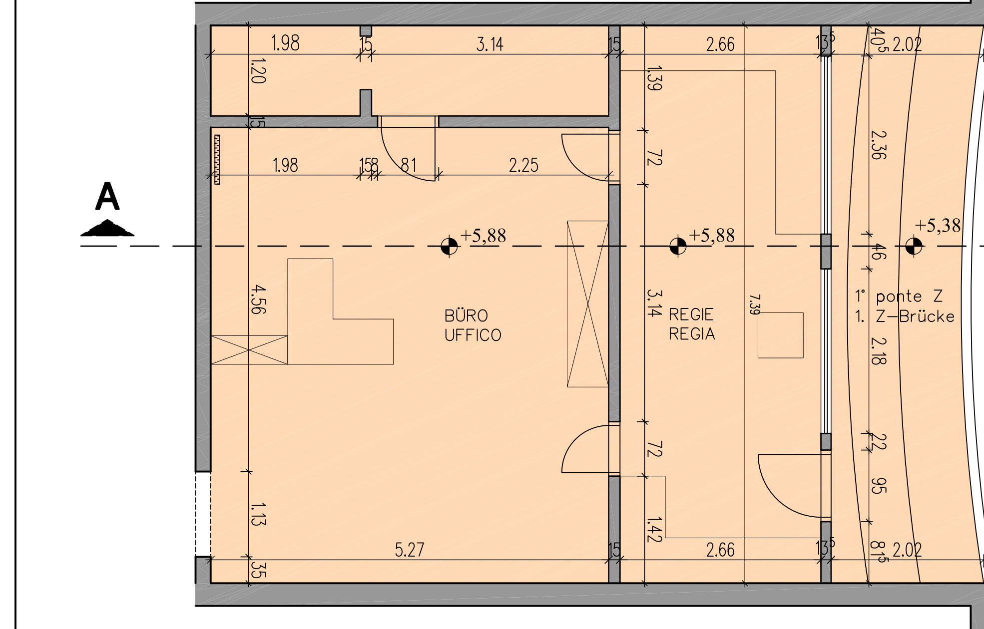
REGIERAUM SALA REGIA 1:50
