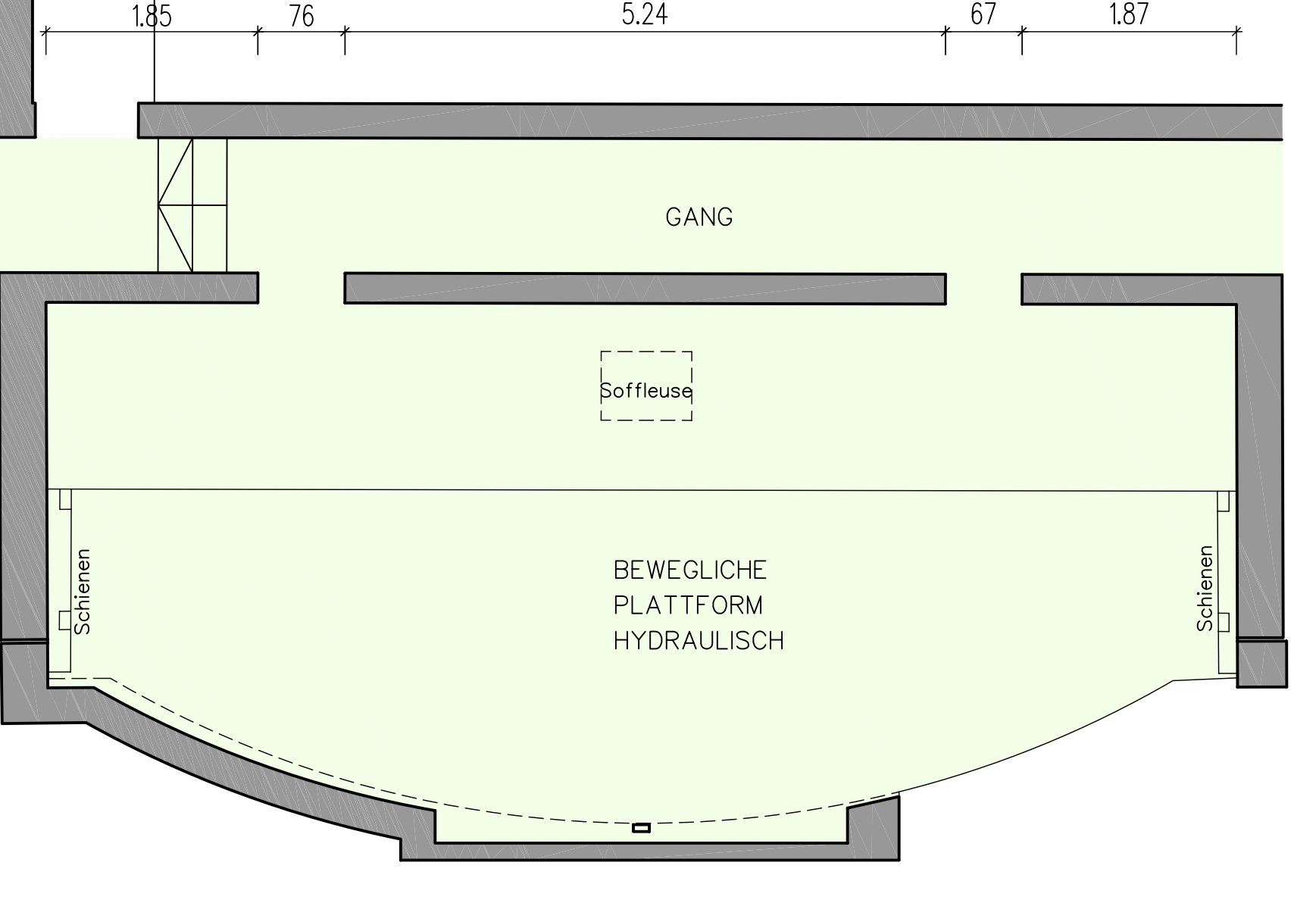
ORCHESTERGRABEN GOLFO MISTICO 1:50
