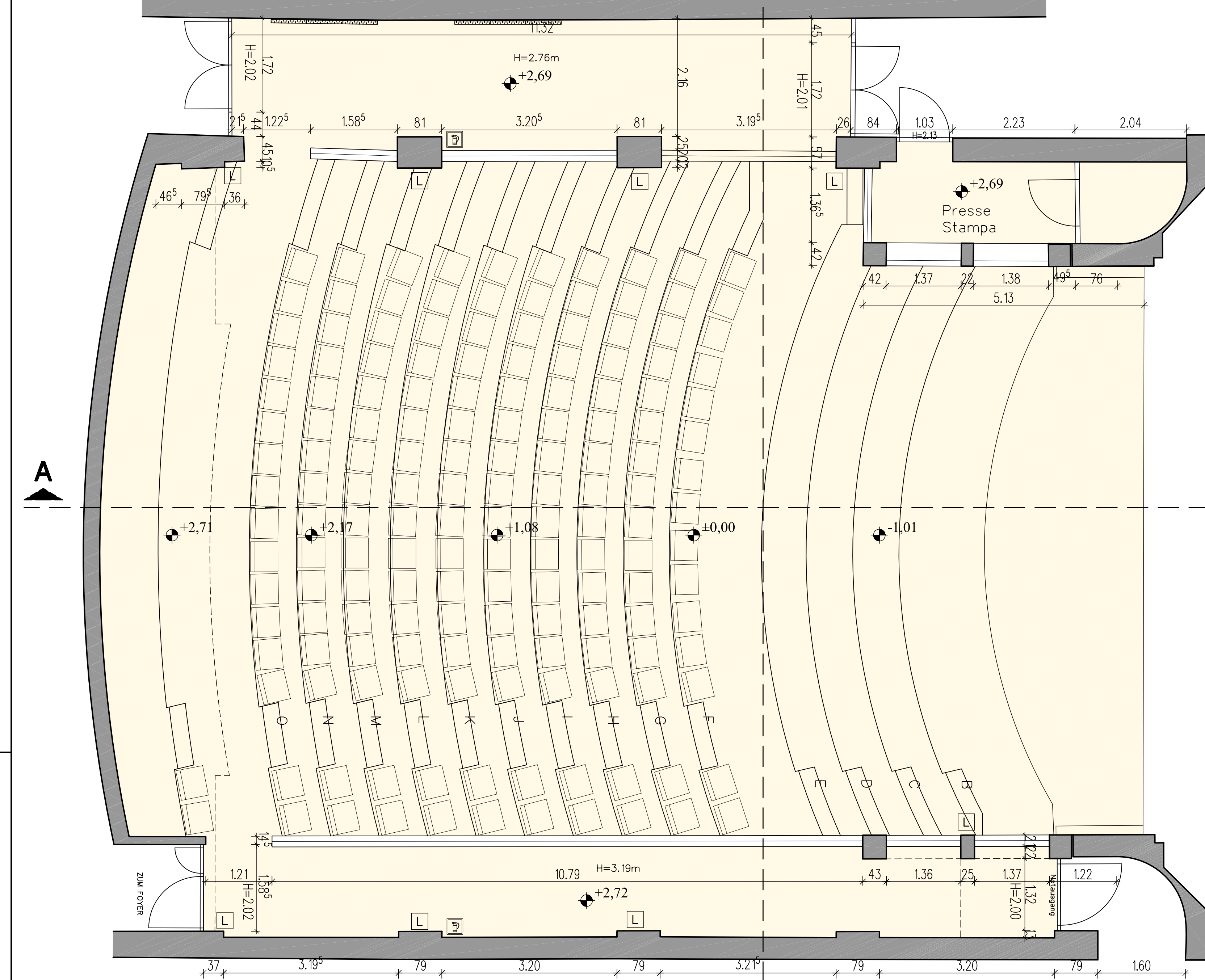
LAGEPLAN ZUSCHAUERRAUM PLANIMETRIA SALA PER I SPETTATORI 1:50
