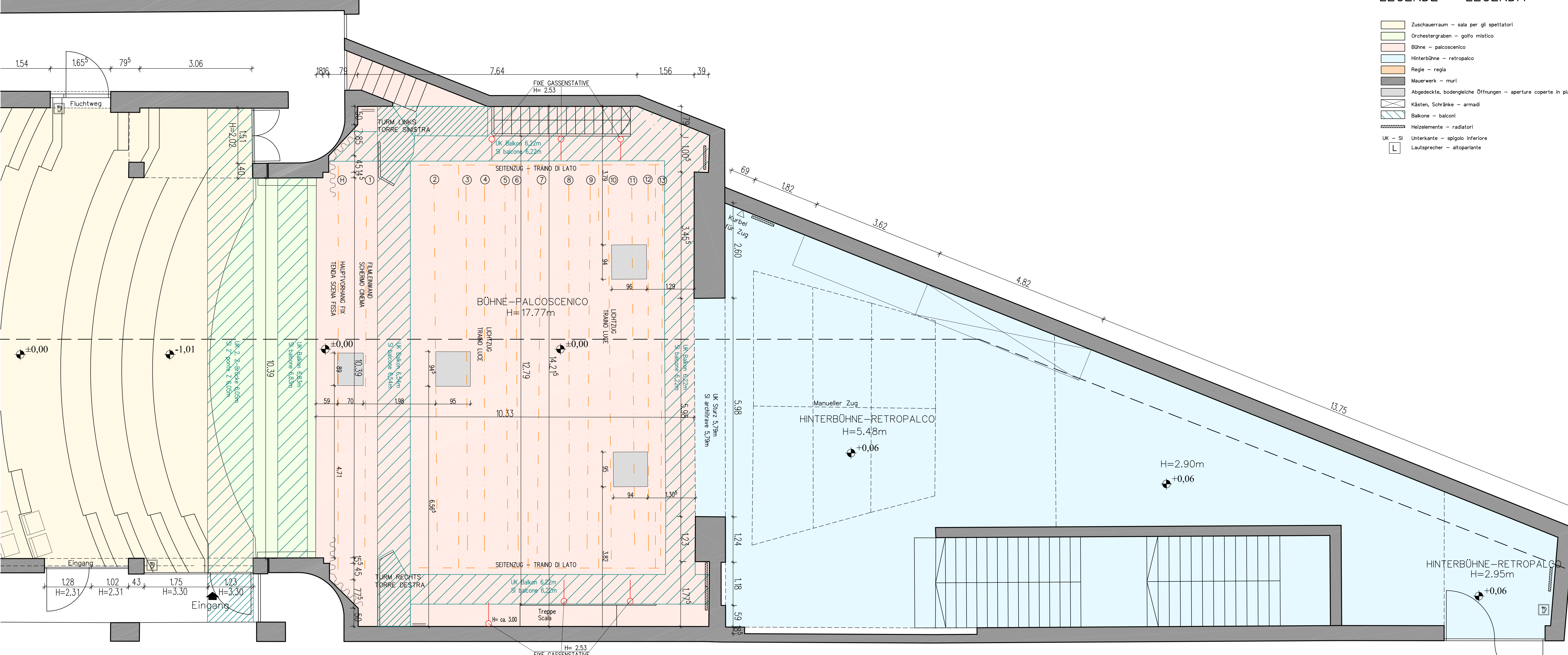
LAGEPLAN BÜHNE PLANIMETRIA PALCOSCENICO 1:50
