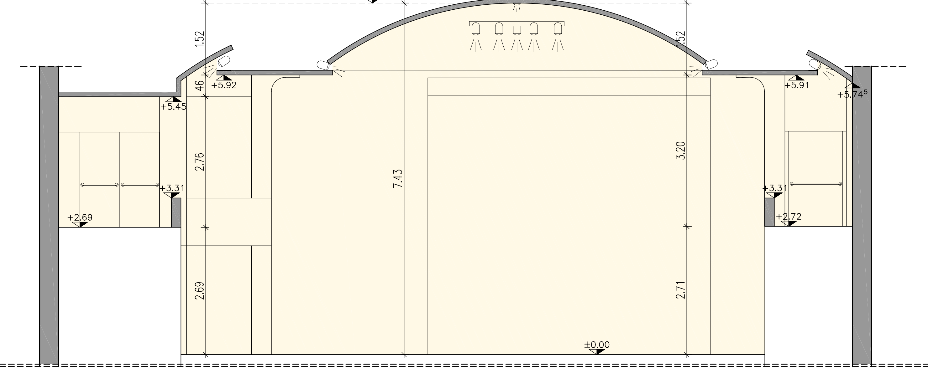
SCHNITT B-B SEZIONE B-B 1:50
